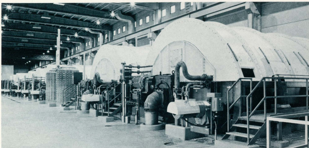
Till Skogsägarnas Industri AB:s nya sulfatfabrik i Värö, som togs i drift 1972, levererade Sunds AB sileri, blekeri samt avvattnings- och balningslinjer. Bilden visar filterplanet i blekeriet med 11 SUND-IMPCO vakuumfilter.
