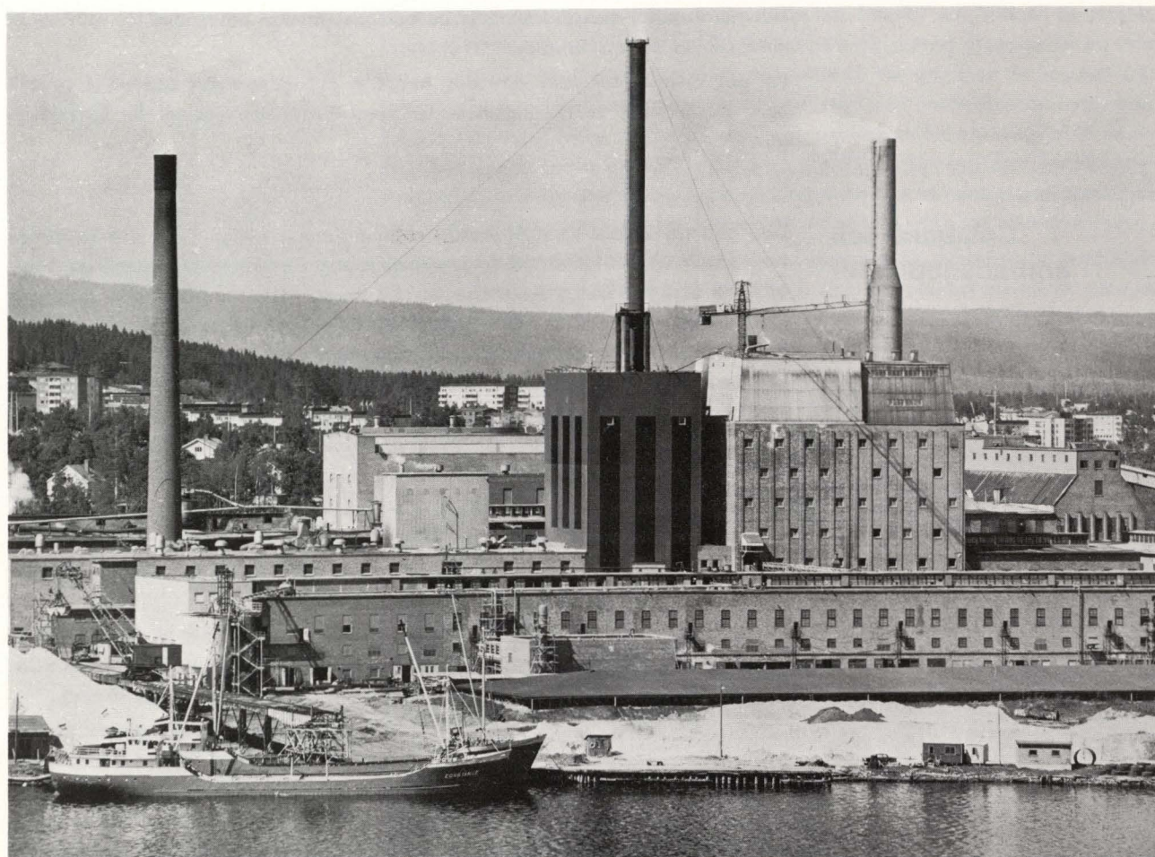
Installation av en ny ångpanna vid Östrands sulfatfabrik har varit den mest betydande investeringen inom cellulosasektorn under 1971. Pannan är inrymd i den nya mörka byggnaden. I förgrunden klorfabriken, vars kapacitet, genom en under 1971 slutförd utbyggnad, ökats från 33.000 ton till 38.000 ton.
